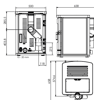
Middenachteraansluitset / Connexion central arrière
