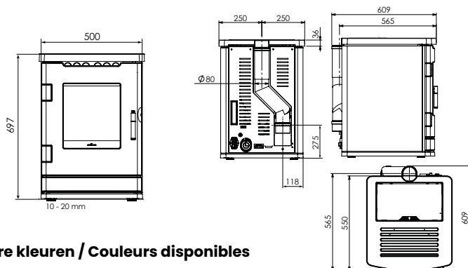
Bovenaansluitset / Connexion supérieure
